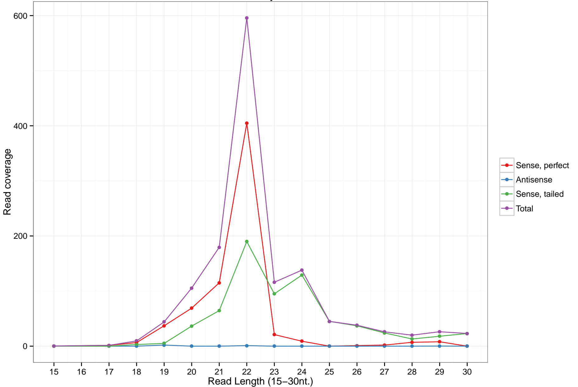
uc009kyr.1
