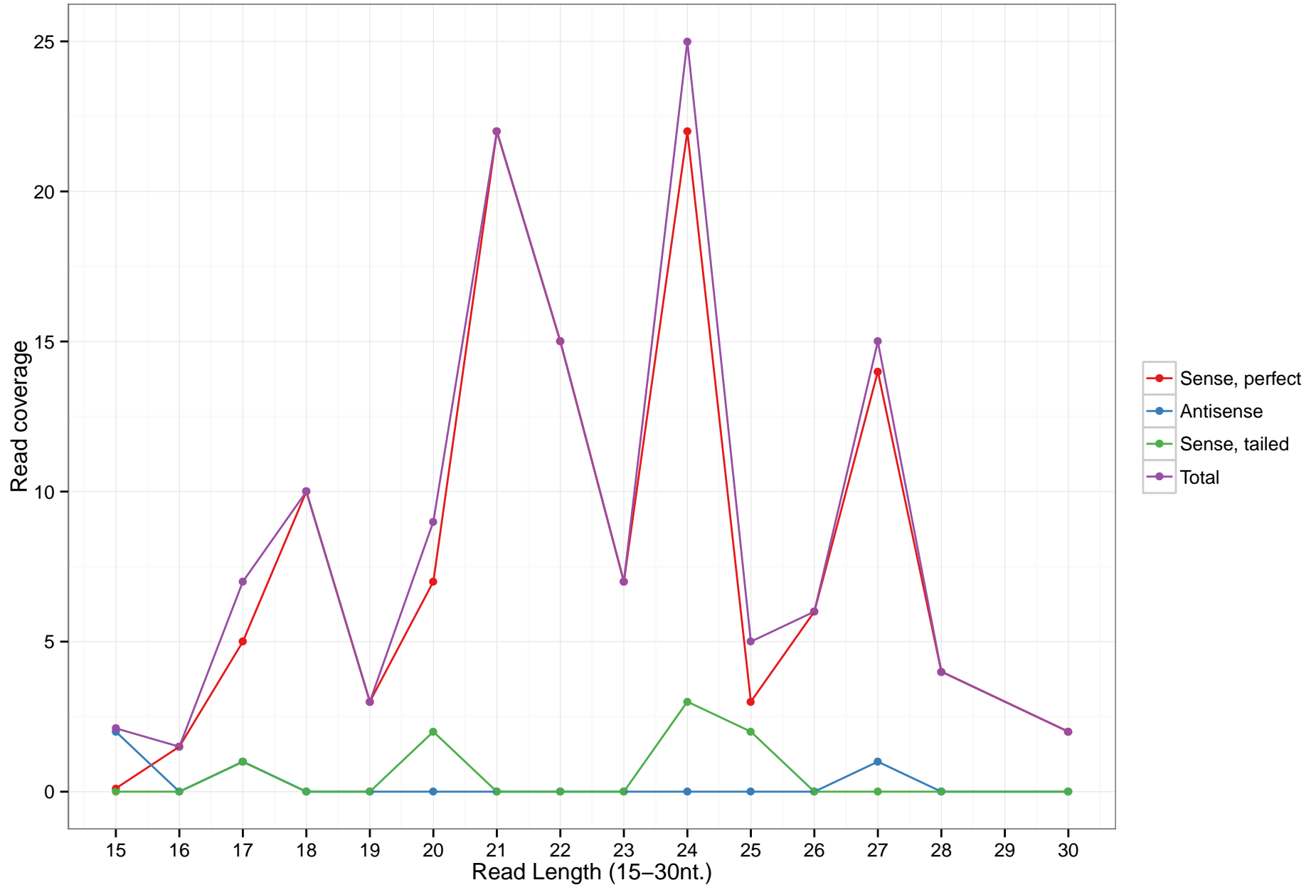
uc008luk.14
