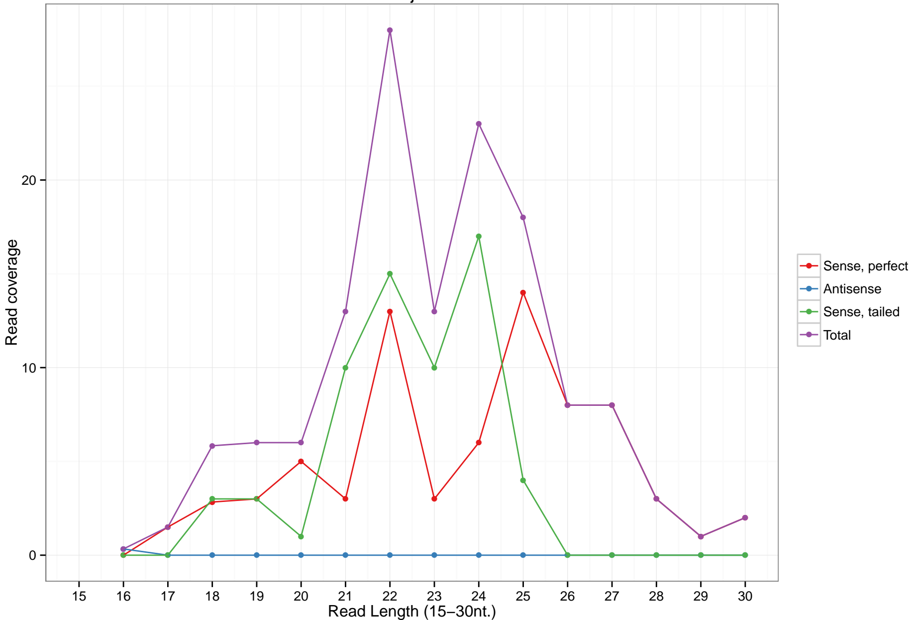
uc007jaw.10
