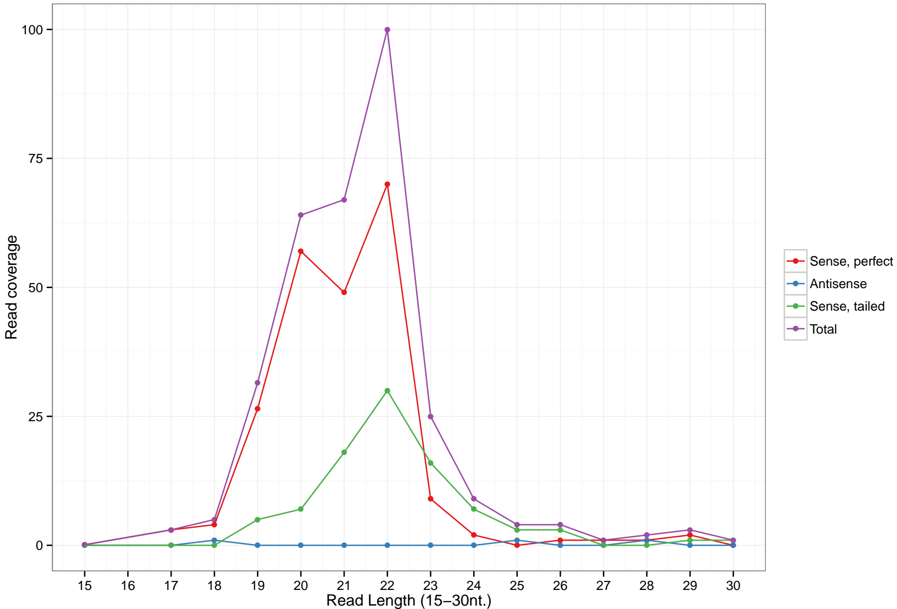
mmu-mir-7082
