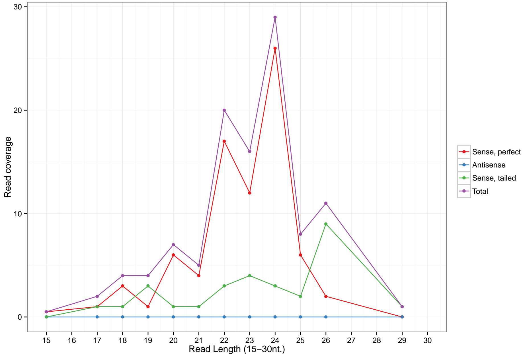
mmu-mir-7037
