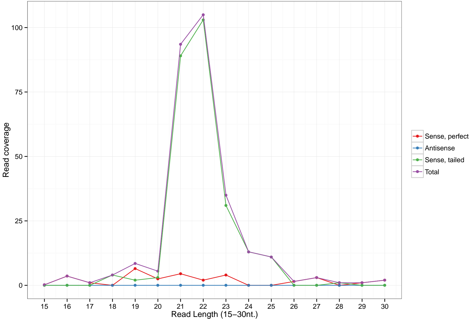
uc011maw.1
