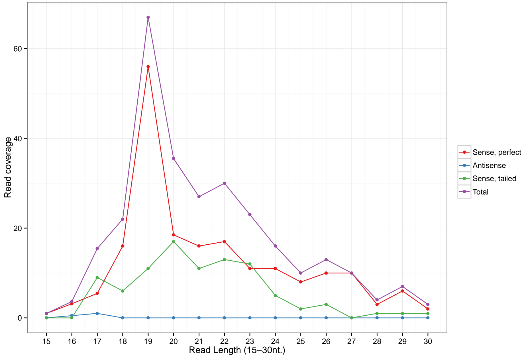
uc004dsn.2
