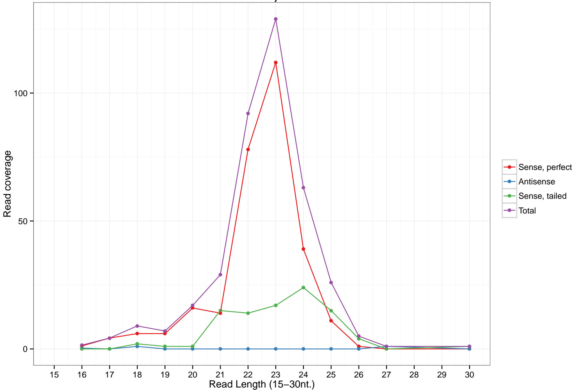
uc003dej.63
