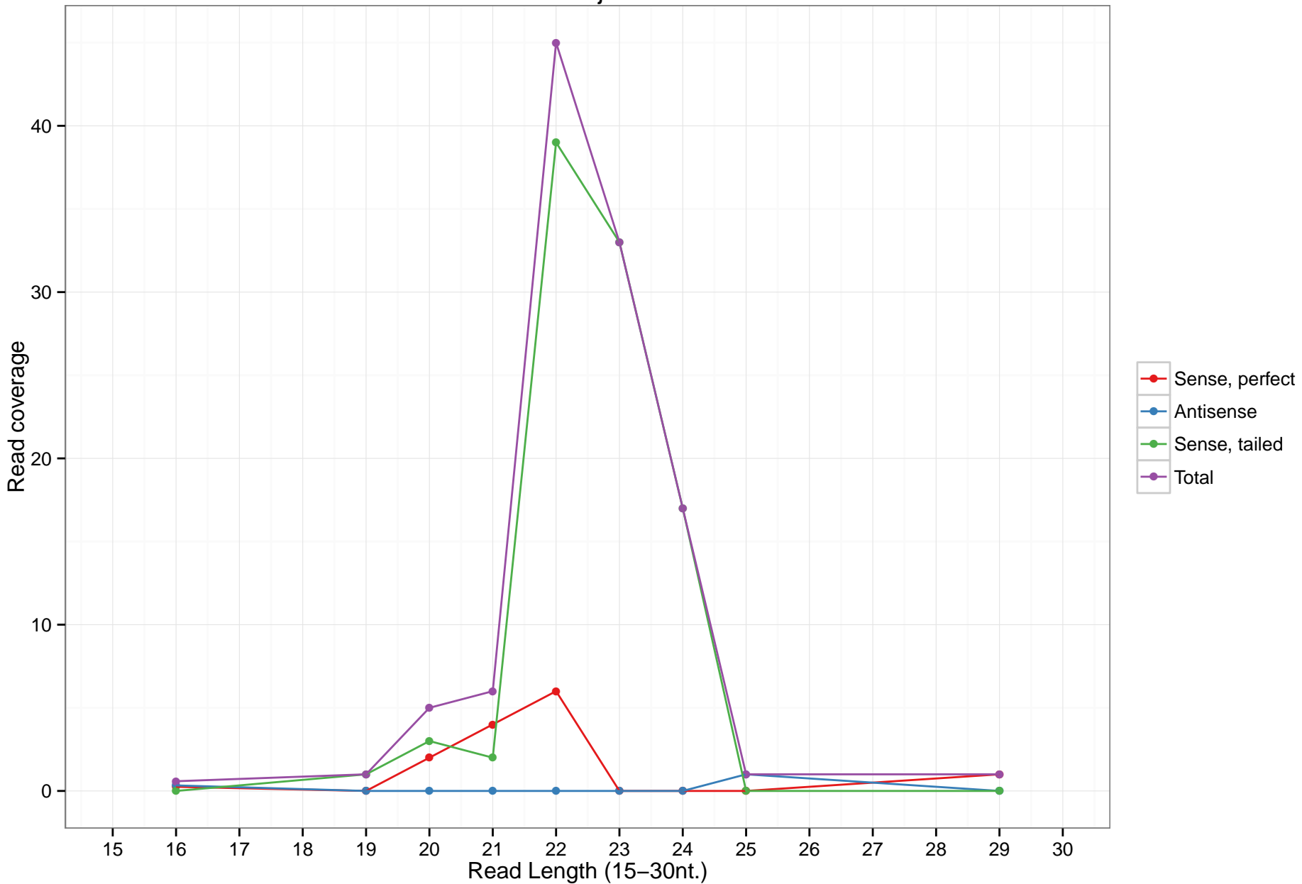
uc001jrd.3
