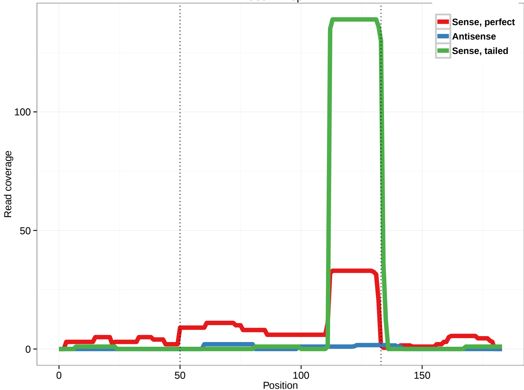
uc011mep.1
