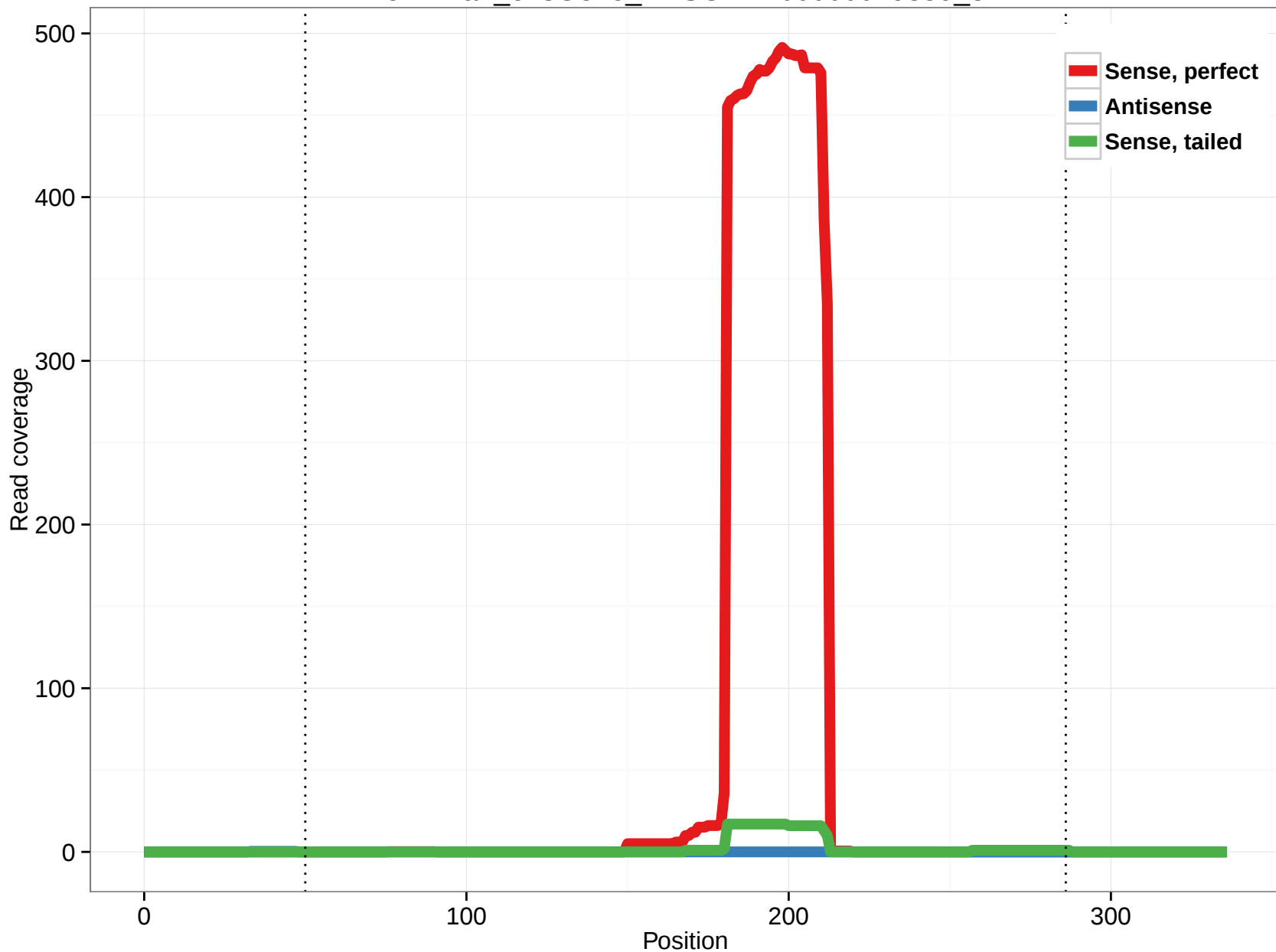
ornAna1_ensGene_ENSOANT00000029859_3
