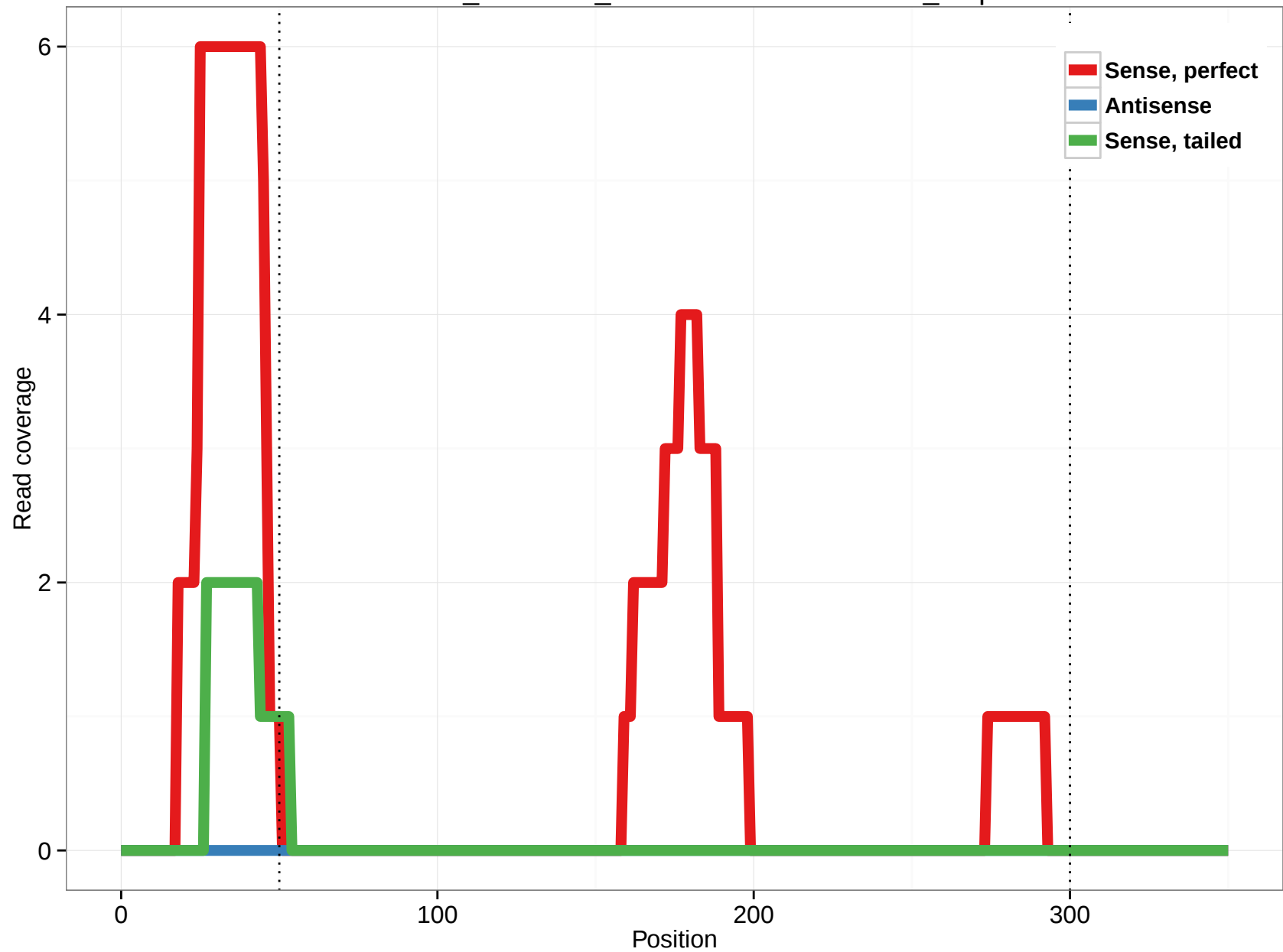
ornAna1_ensGene_ENSOANT00000024378_7.5p
