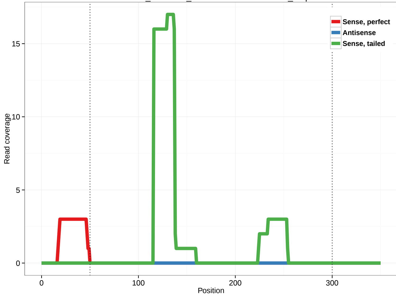
ornAna1_ensGene_ENSOANT00000022561_7.5p
