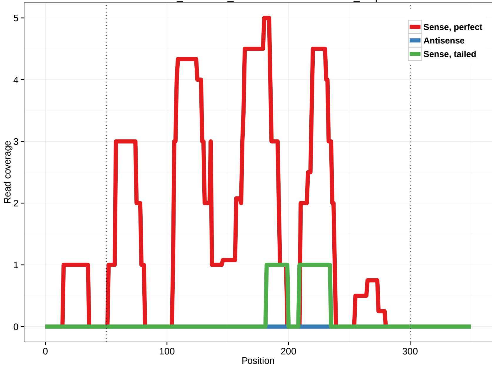
ornAna1_ensGene_ENSOANT00000022537_7.5p
