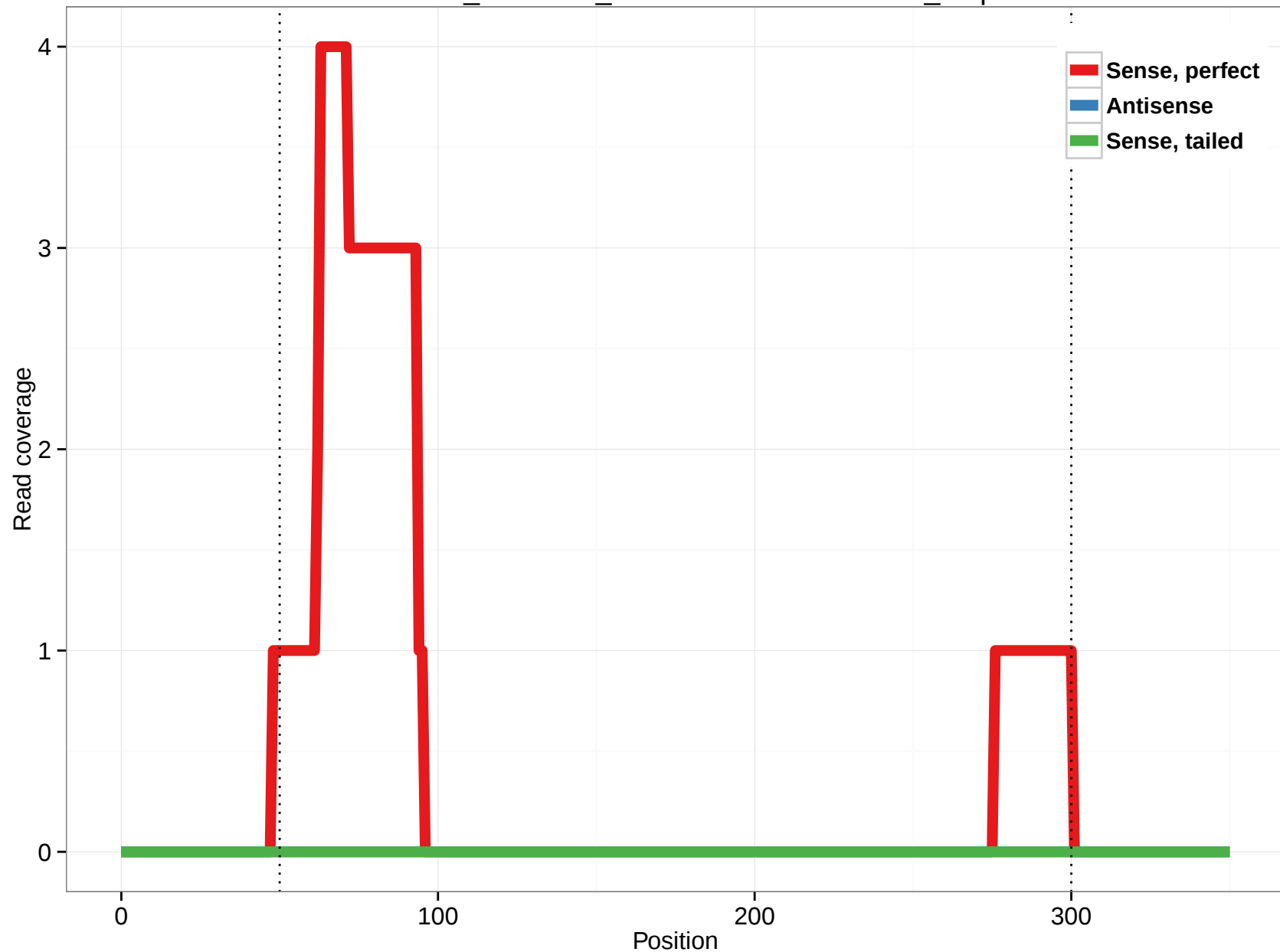
ornAna1_ensGene_ENSOANT00000022252_1.3p
