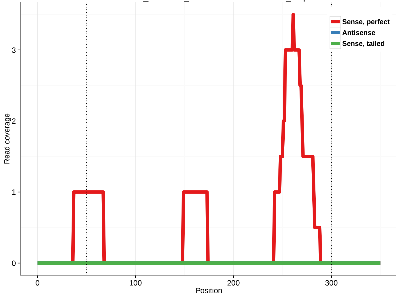
ornAna1_ensGene_ENSOANT00000019835_2.5p
