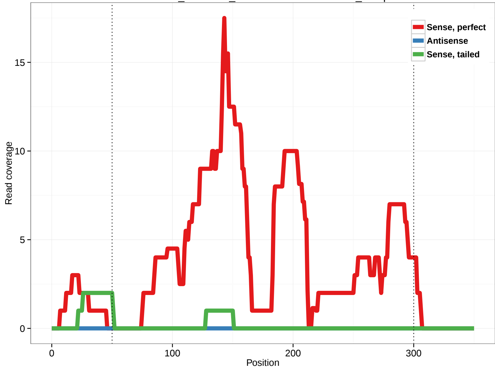
ornAna1_ensGene_ENSOANT00000017739_30.5p
