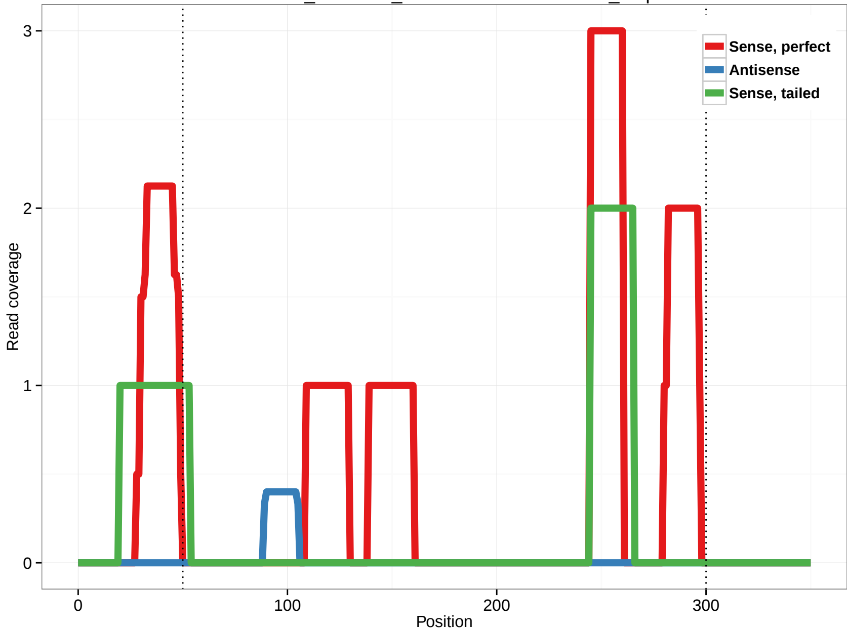
ornAna1_ensGene_ENSOANT00000017128_9.5p
