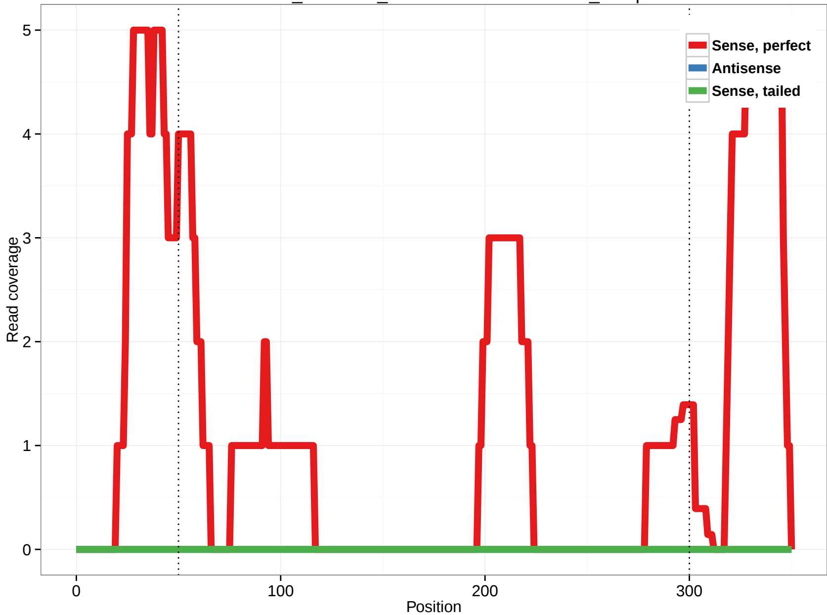
ornAna1_ensGene_ENSOANT00000016750_10.5p
