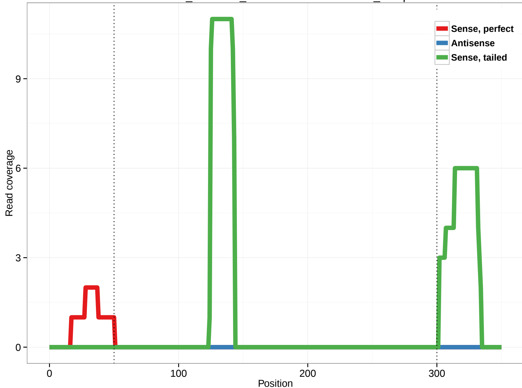
ornAna1_ensGene_ENSOANT00000016422_10.5p
