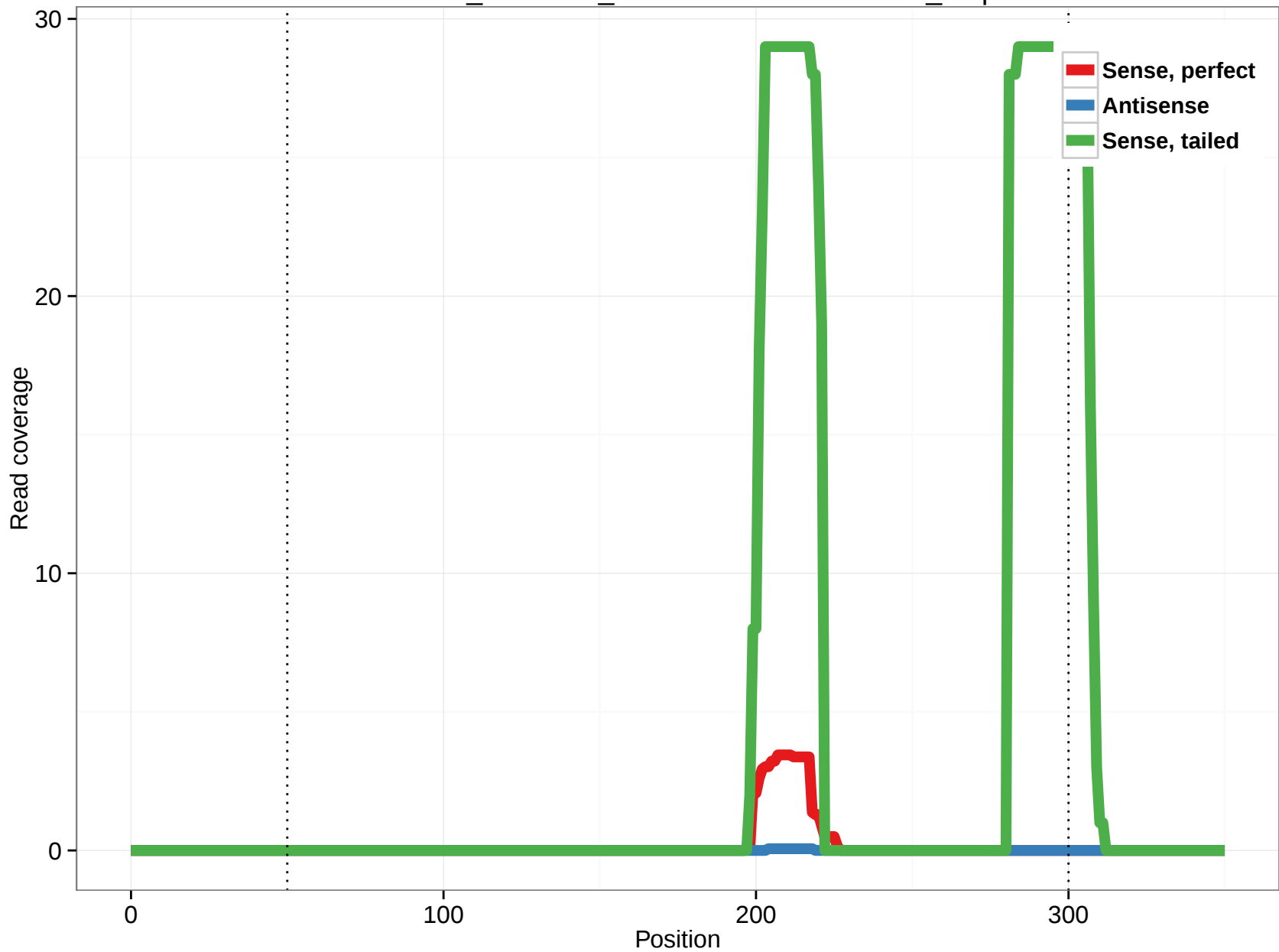
ornAna1_ensGene_ENSOANT00000012532_1.5p
