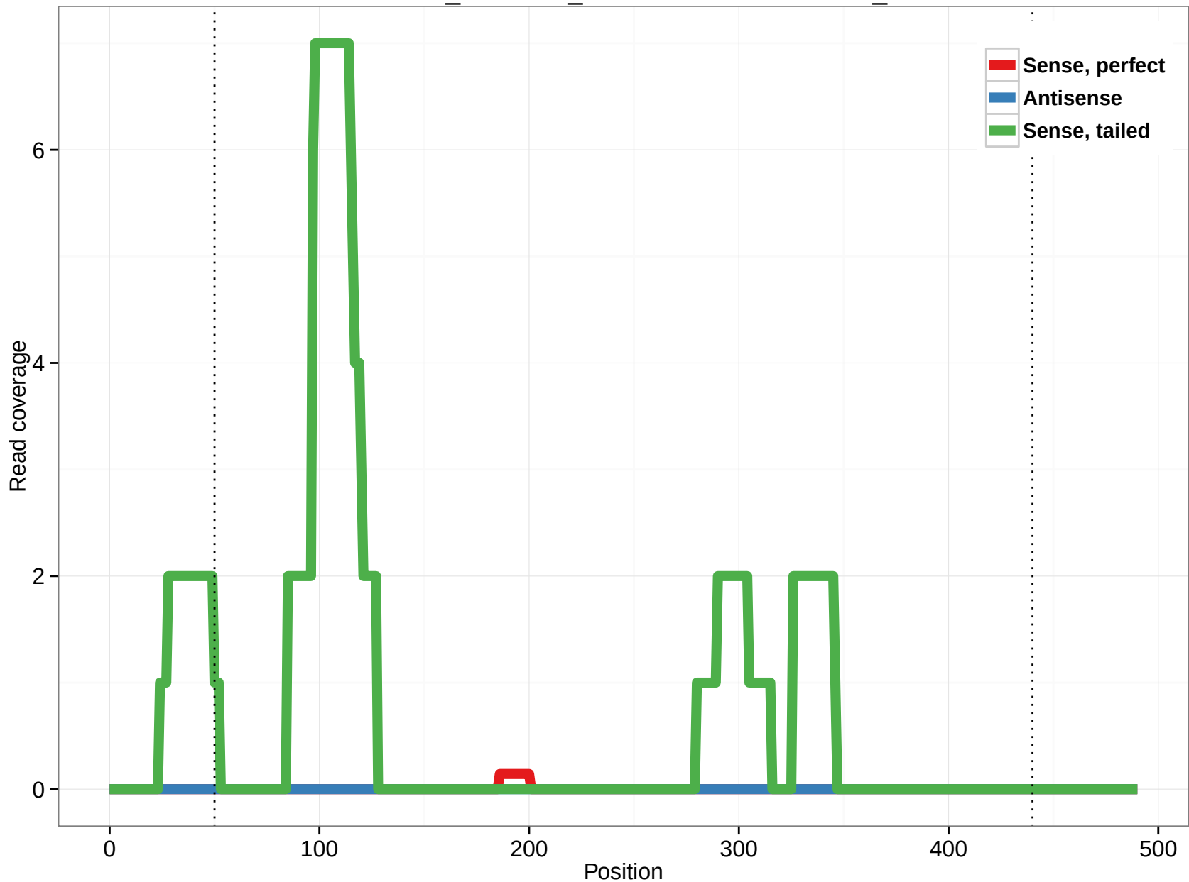
ornAna1_ensGene_ENSOANT00000012394_0
