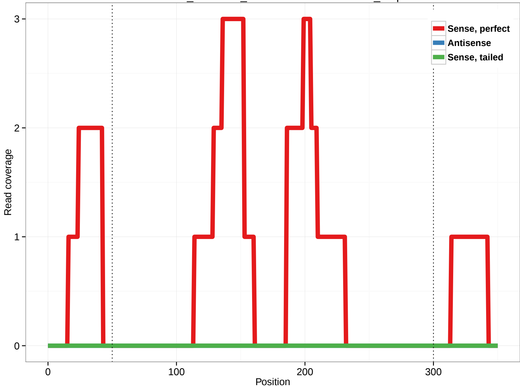
ornAna1_ensGene_ENSOANT00000011816_8.5p
