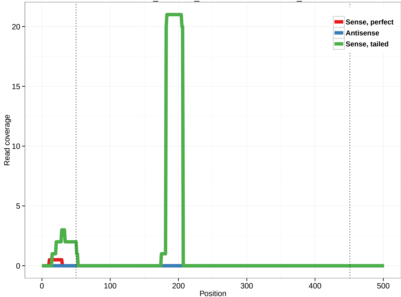
ornAna1_ensGene_ENSOANT00000010256_5
