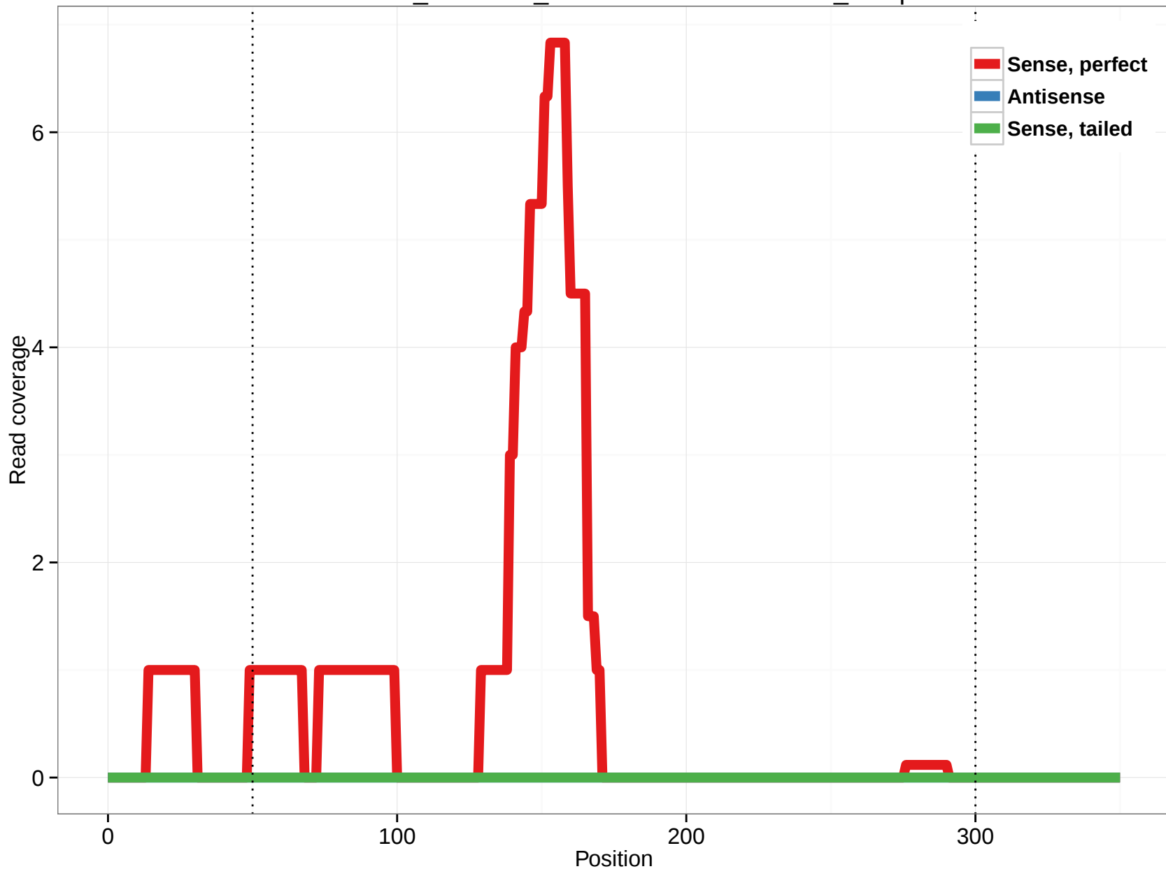
ornAna1_ensGene_ENSOANT00000009352_11.5p
