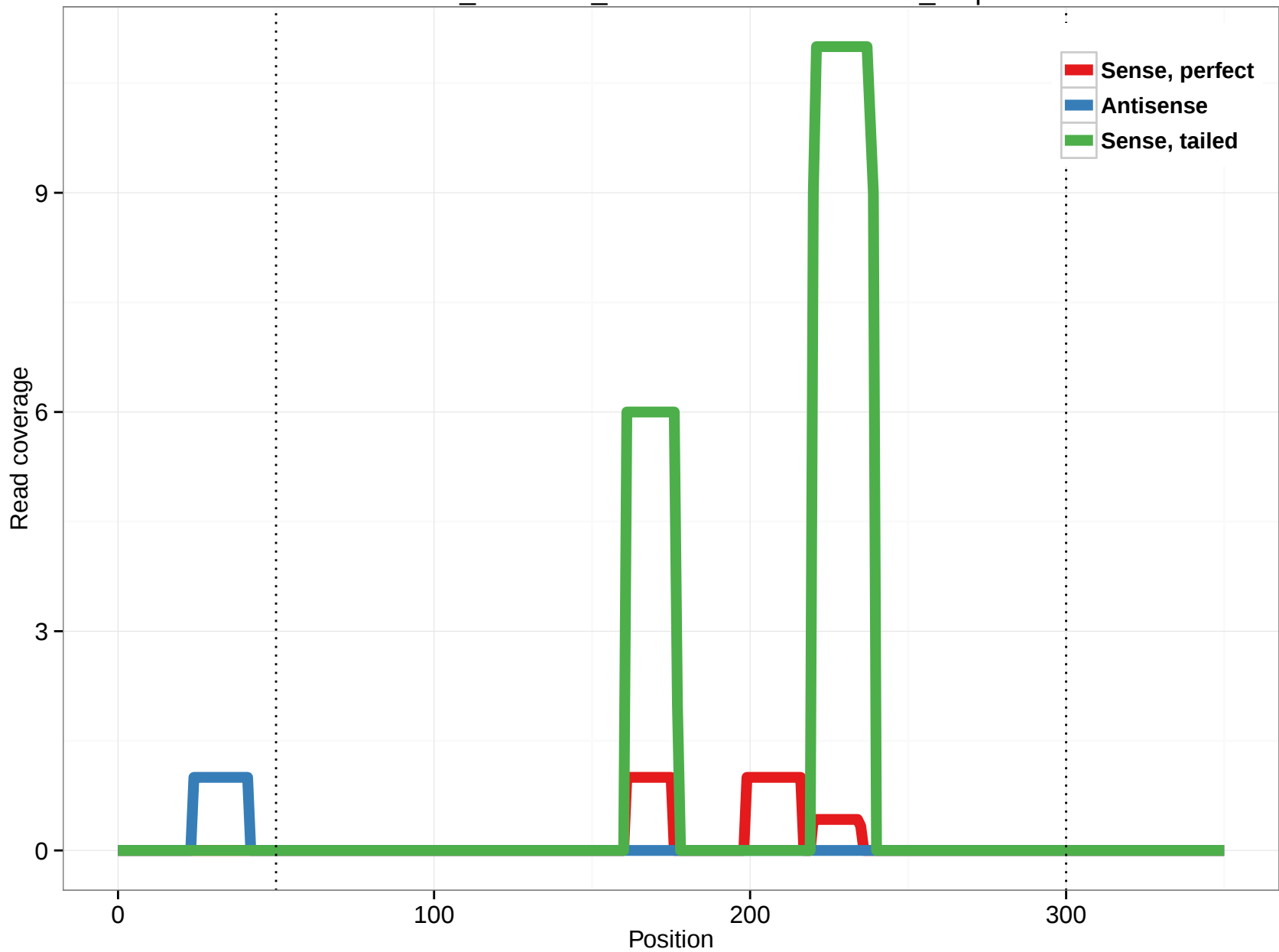
ornAna1_ensGene_ENSOANT00000009294_9.5p
