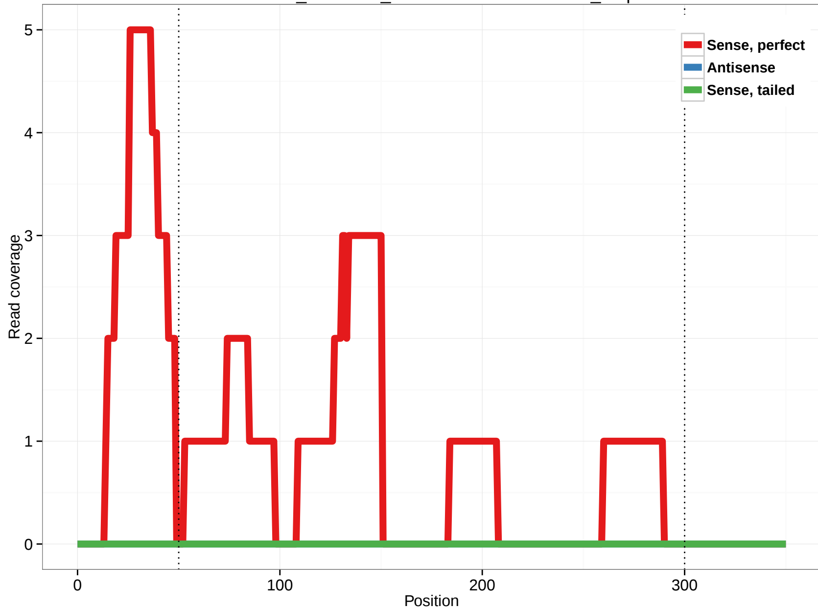
ornAna1_ensGene_ENSOANT00000007161_4.5p
