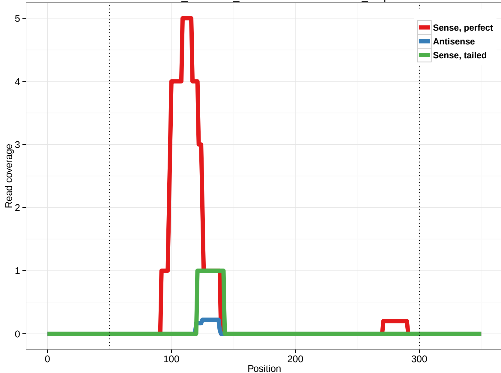
ornAna1_ensGene_ENSOANT00000004905_9.5p
