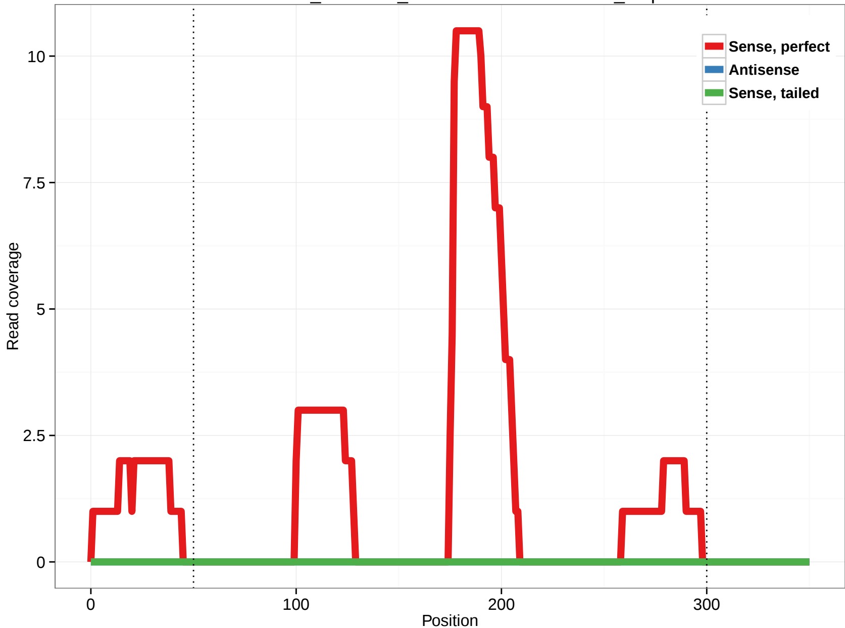
ornAna1_ensGene_ENSOANT00000002758_7.5p
