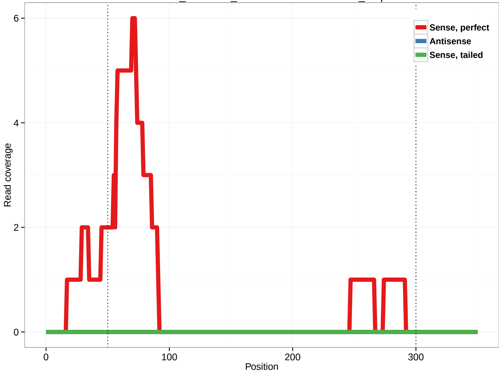
ornAna1_ensGene_ENSOANT00000002481_9.5p
