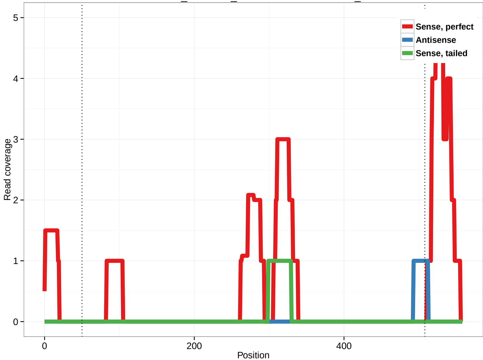
ornAna1_ensGene_ENSOANT00000001549_2
