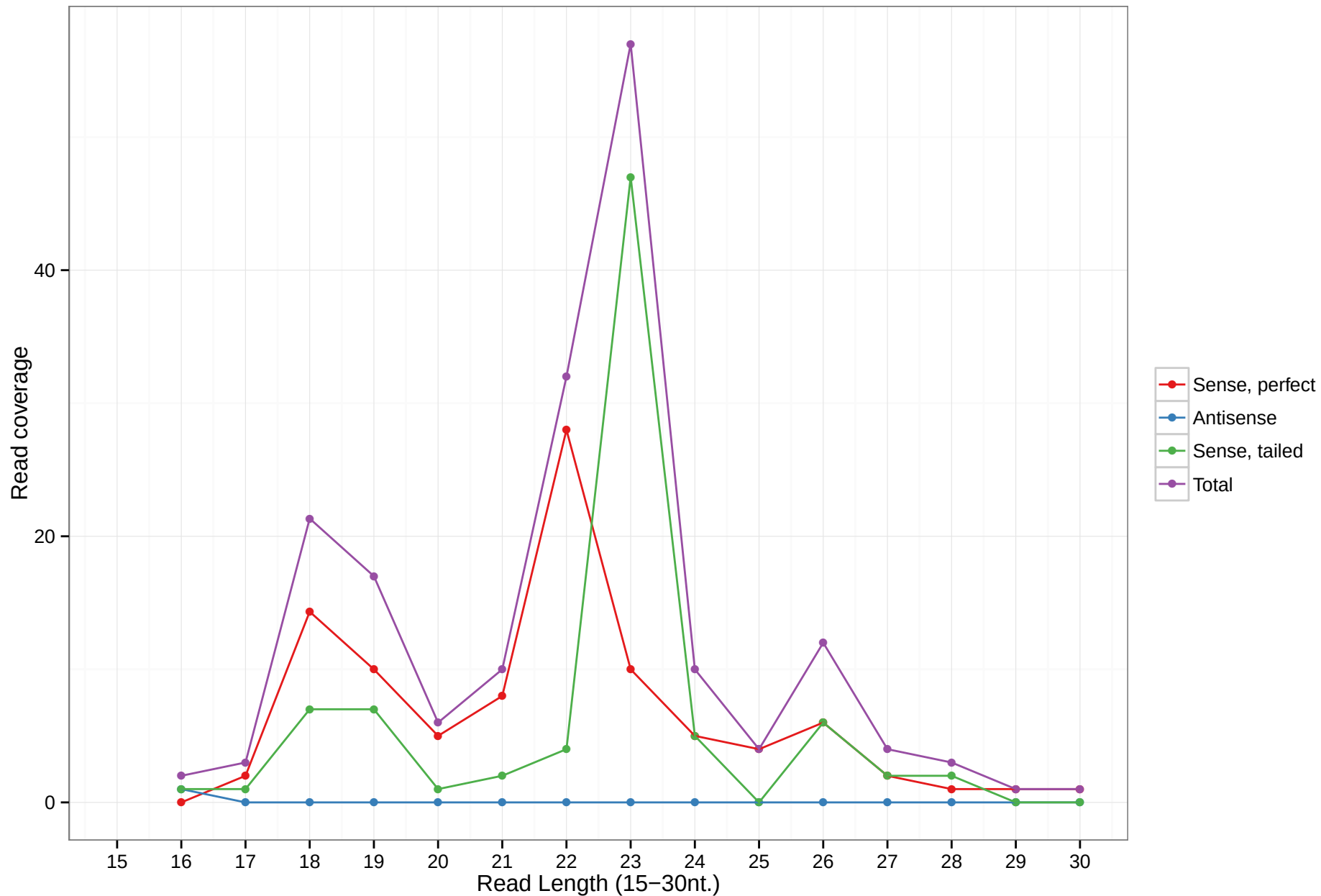
uc009acd.3
