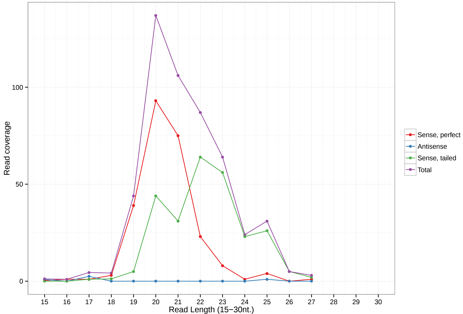
uc008wrm.0
