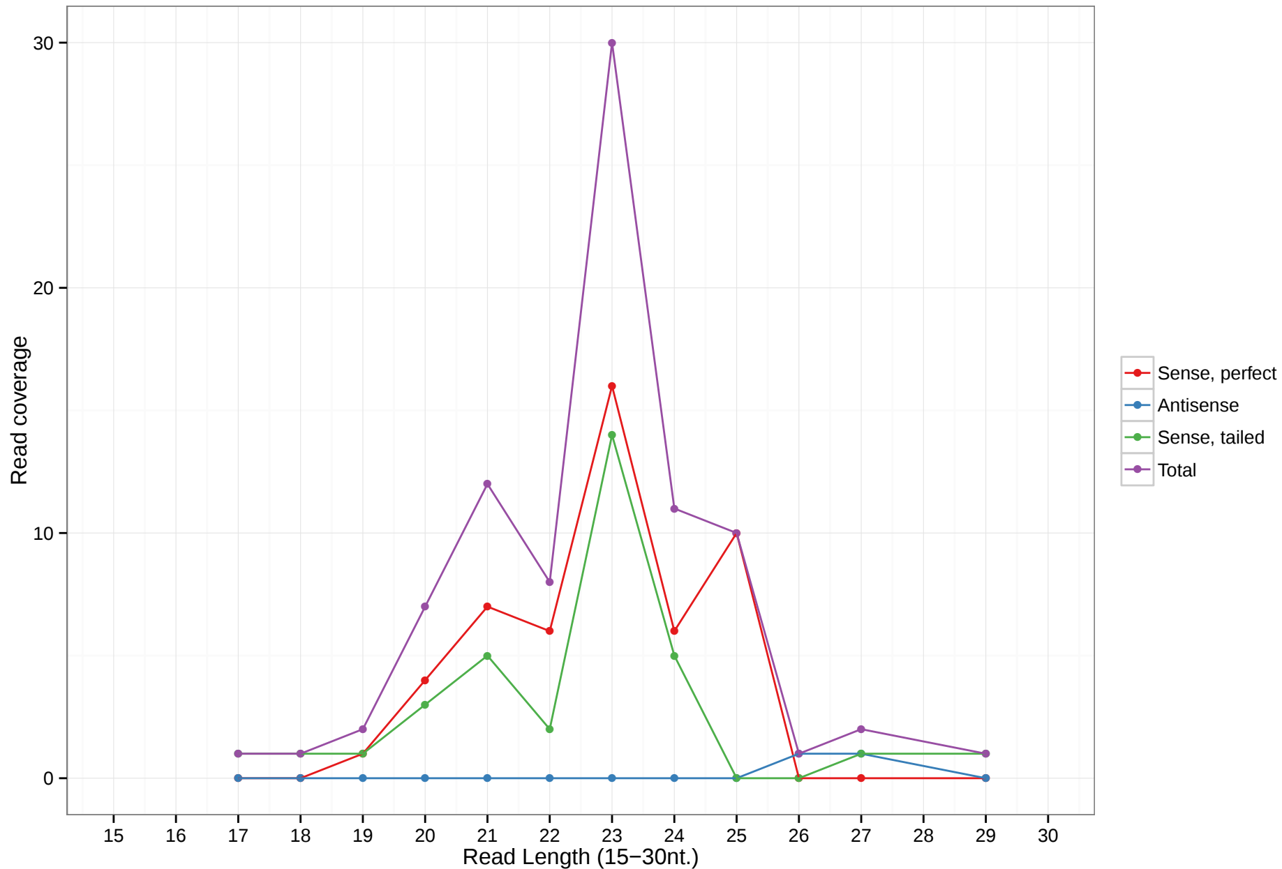
uc008bco.4
