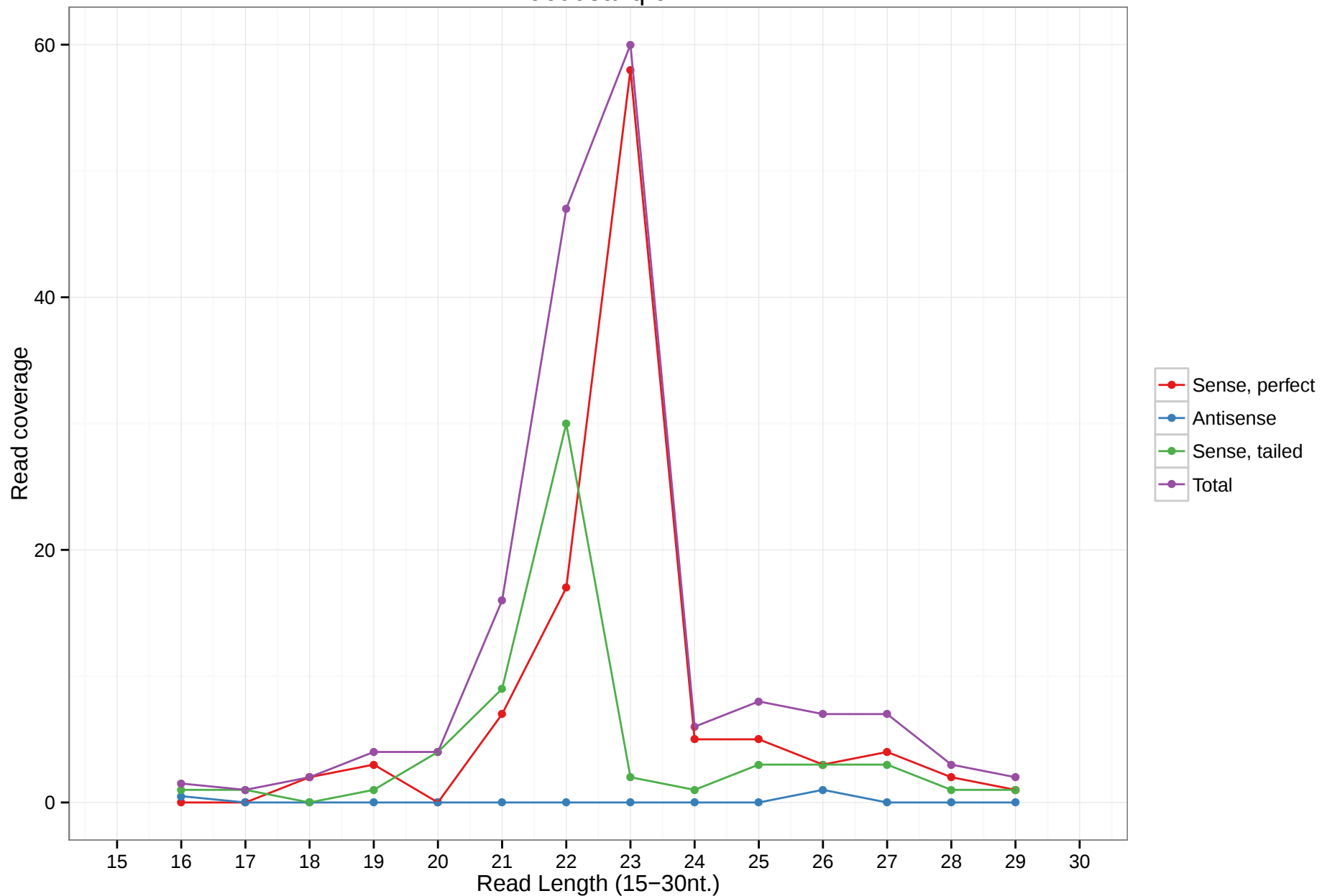
uc008azq.6
