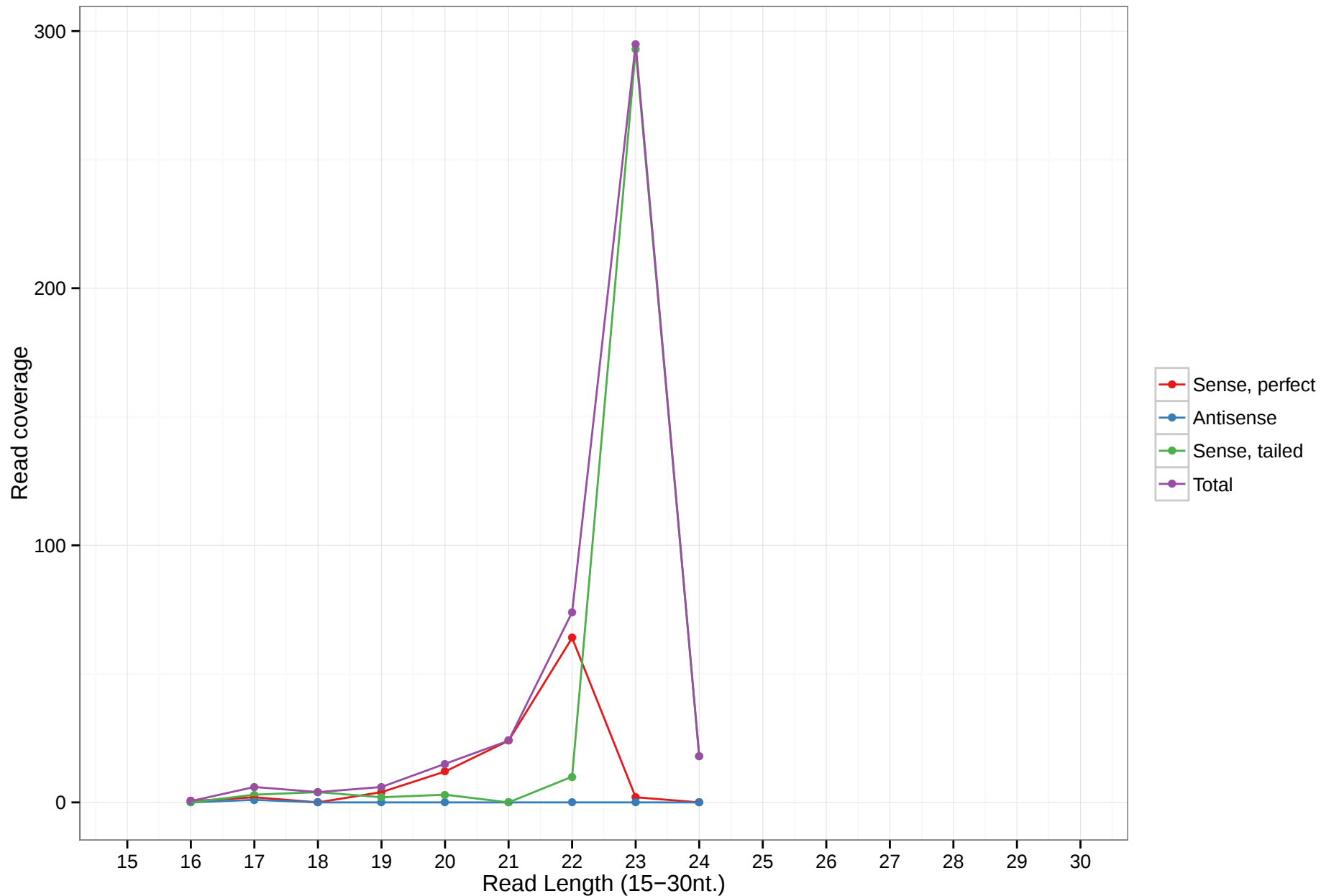
uc007wxs.1
