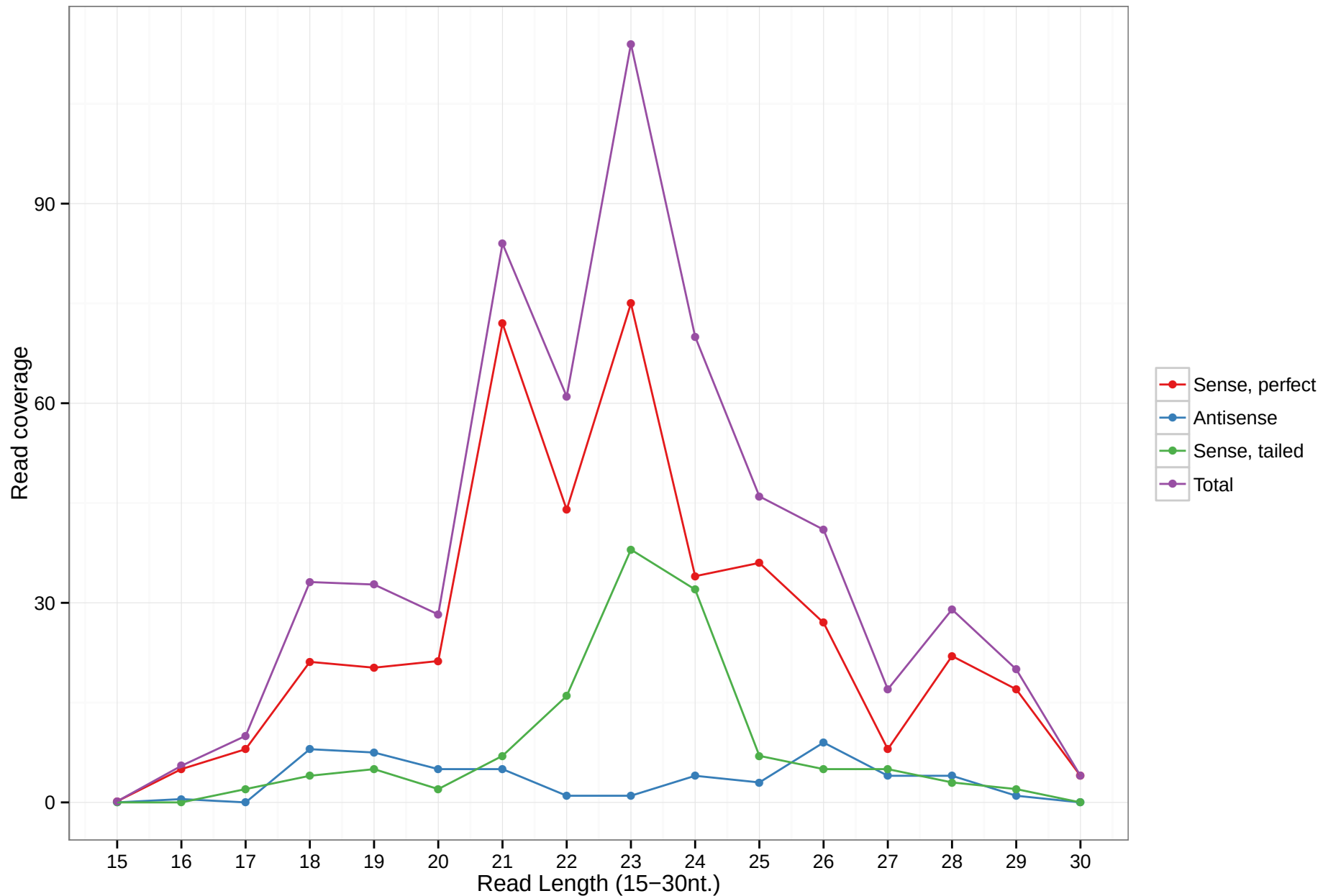
uc007ldu.20
