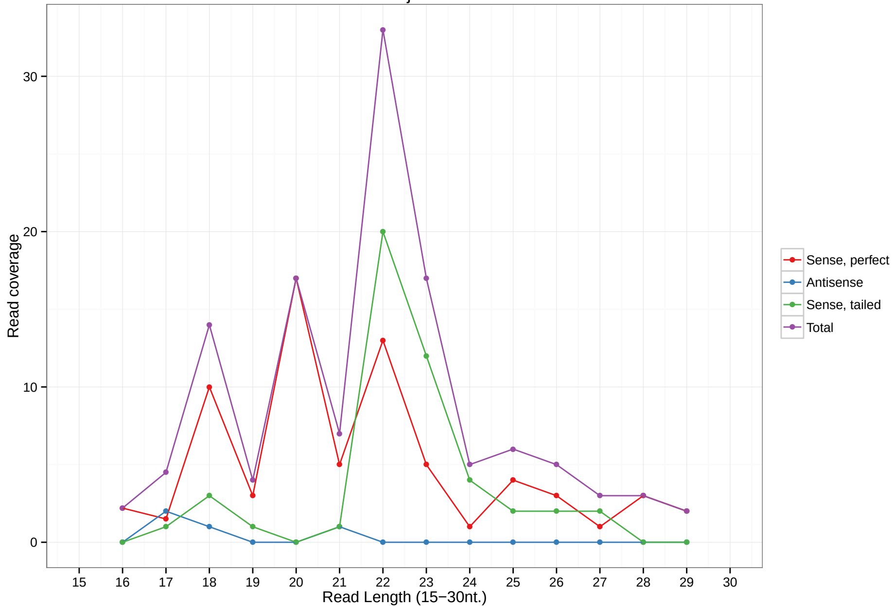
uc007jhm.3
