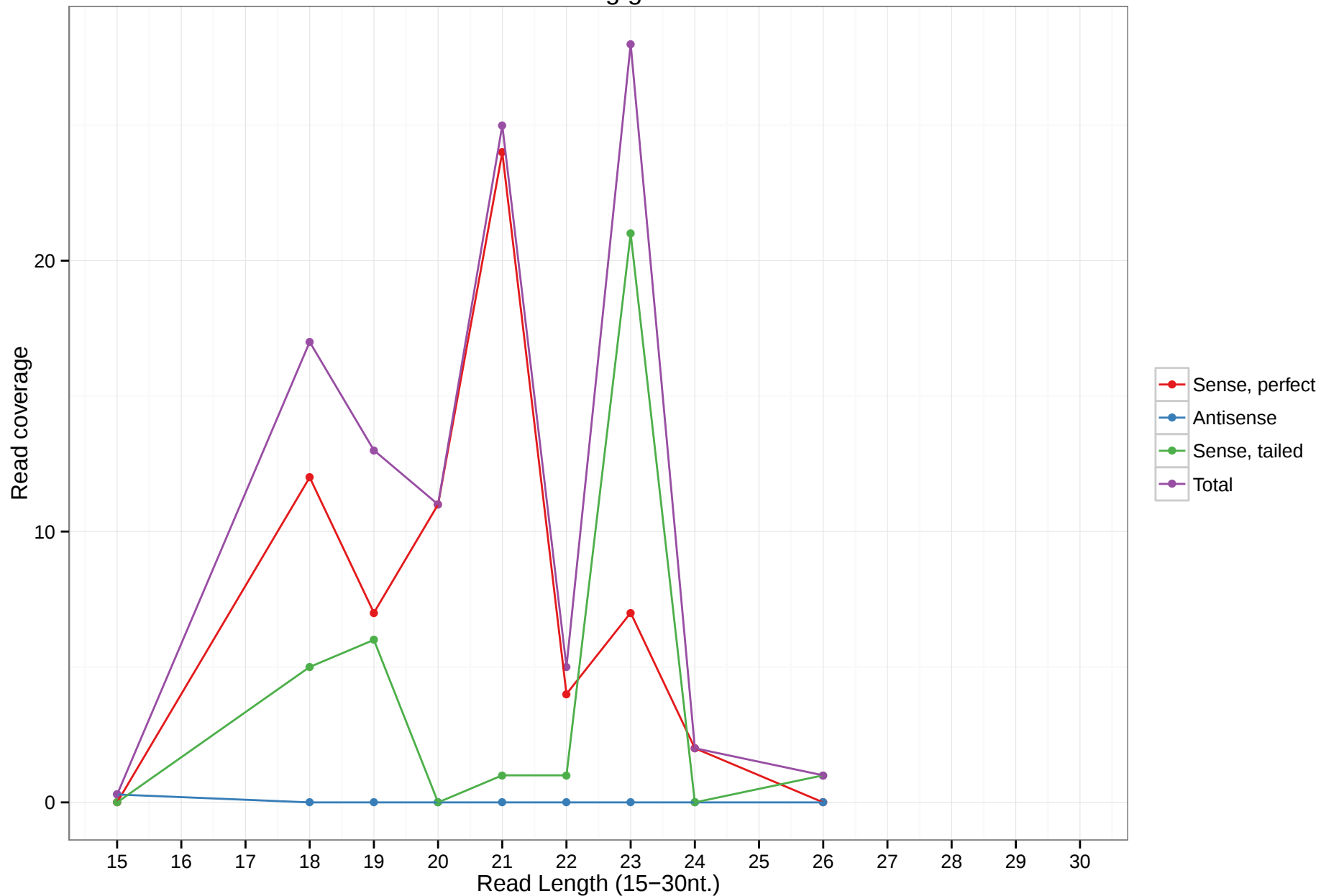
uc007gtg.2
