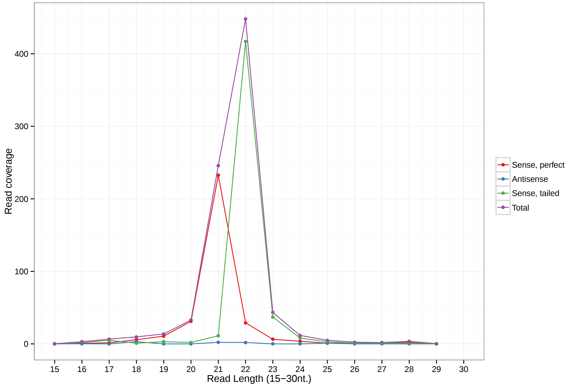
mmu-mir-7093
