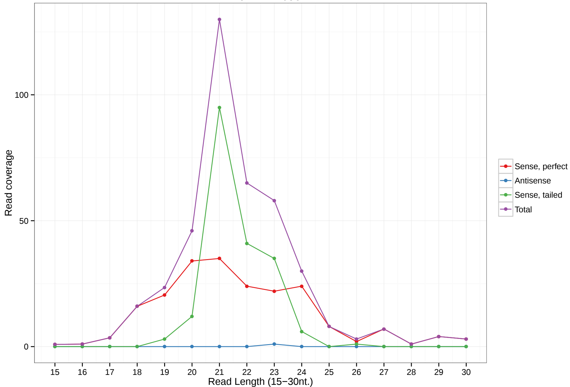
mmu-mir-7090
