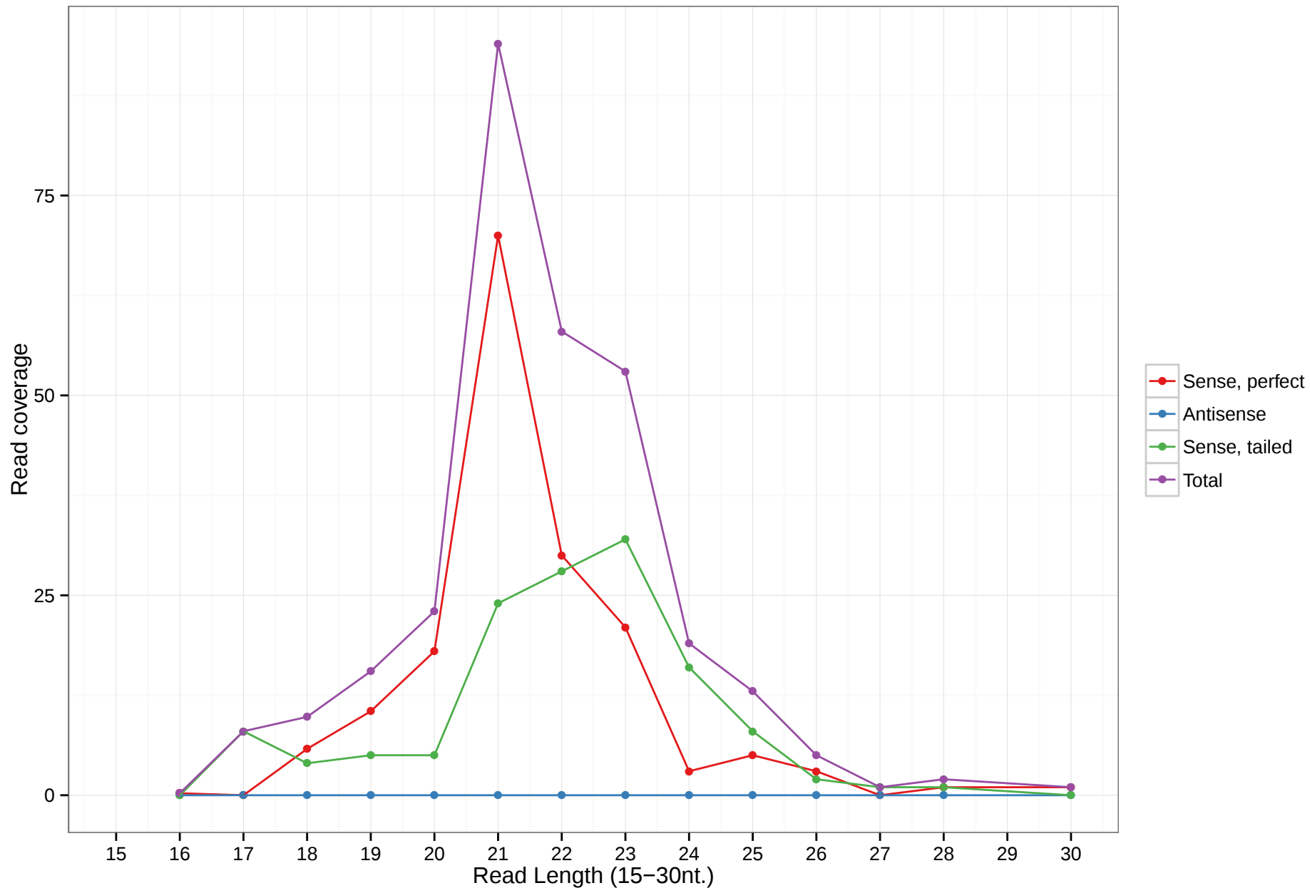
mmu-mir-7087
