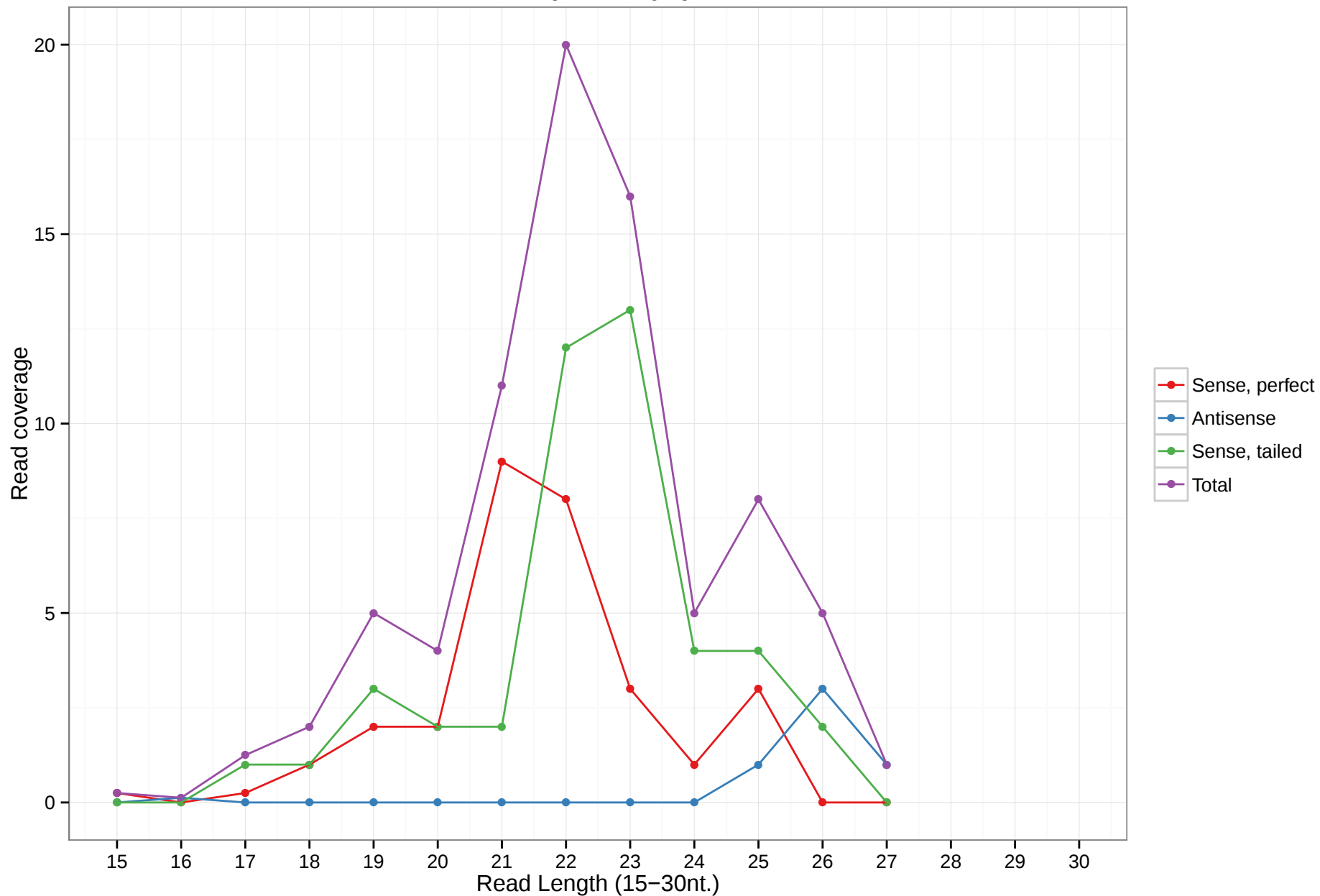
mmu-mir-7076
