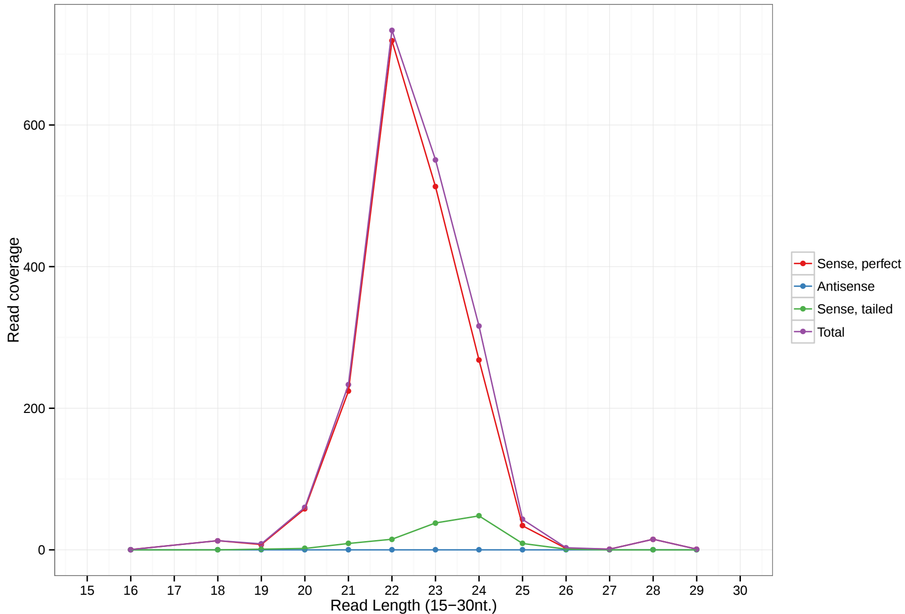
mmu-mir-7073
