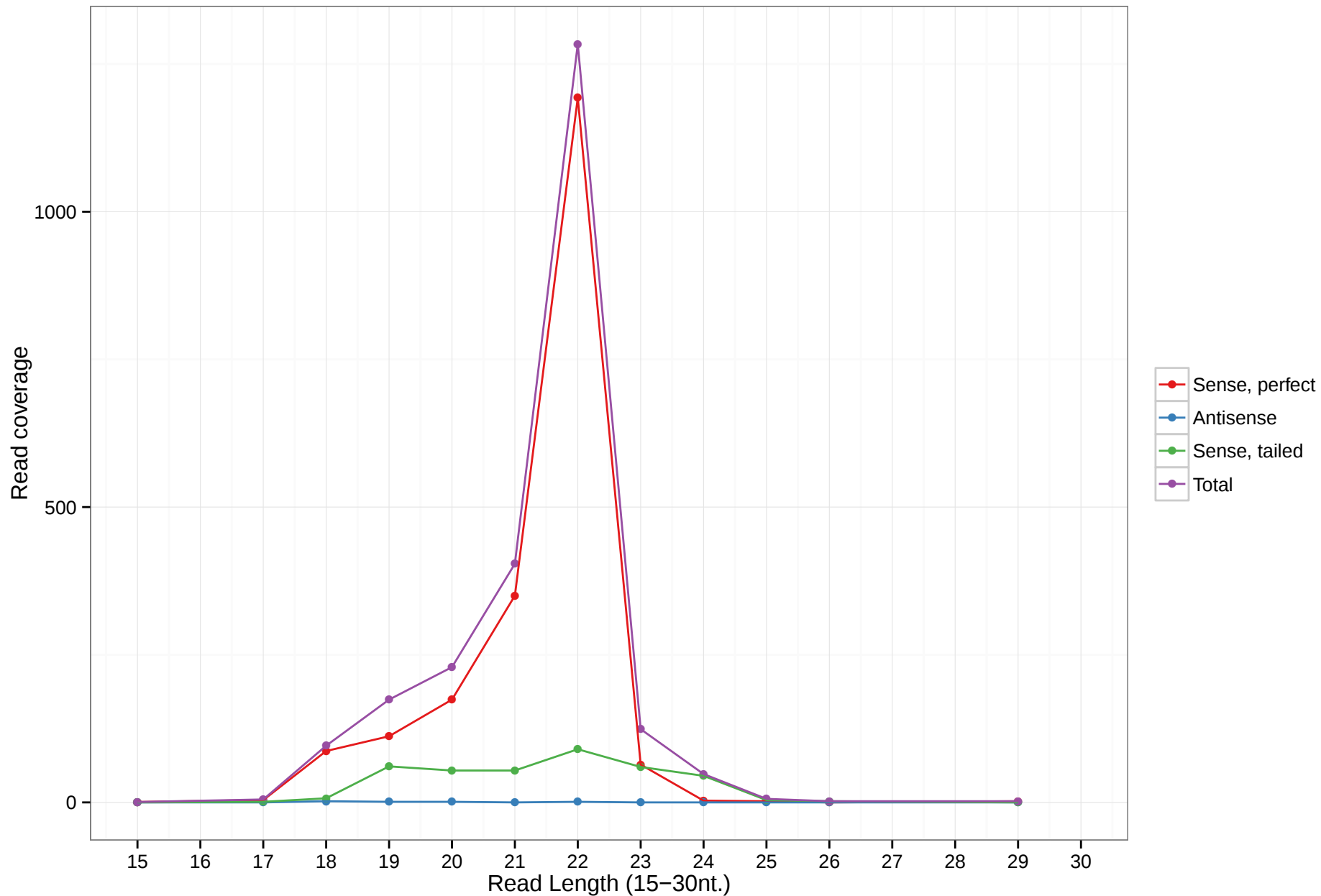
mmu-mir-7059
