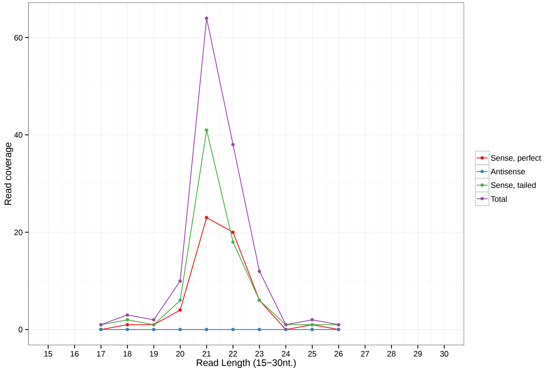
mmu-mir-7057
