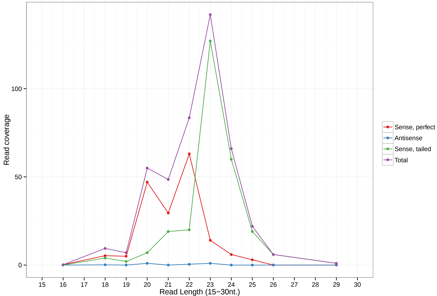
mmu-mir-7056
