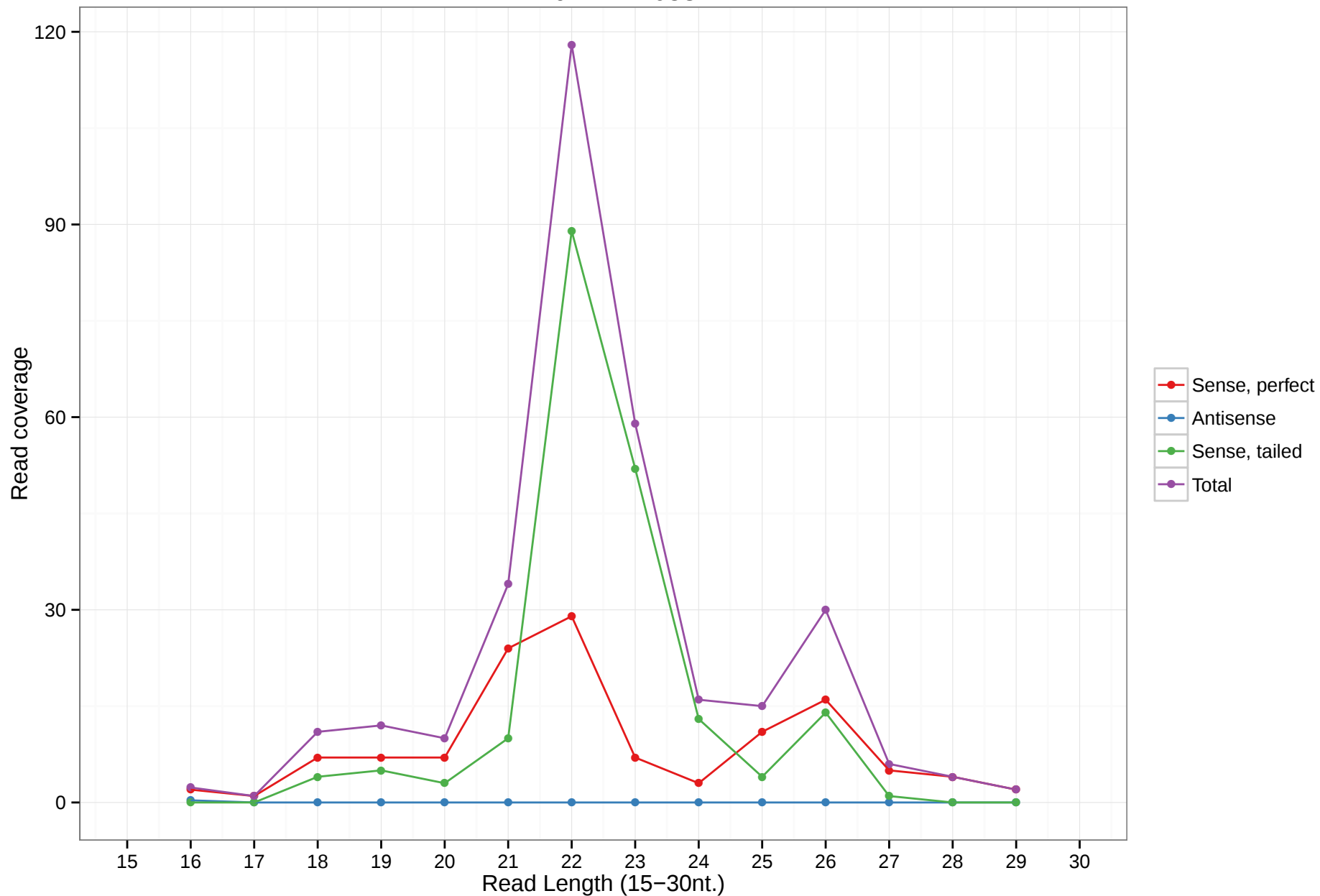
mmu-mir-7053
