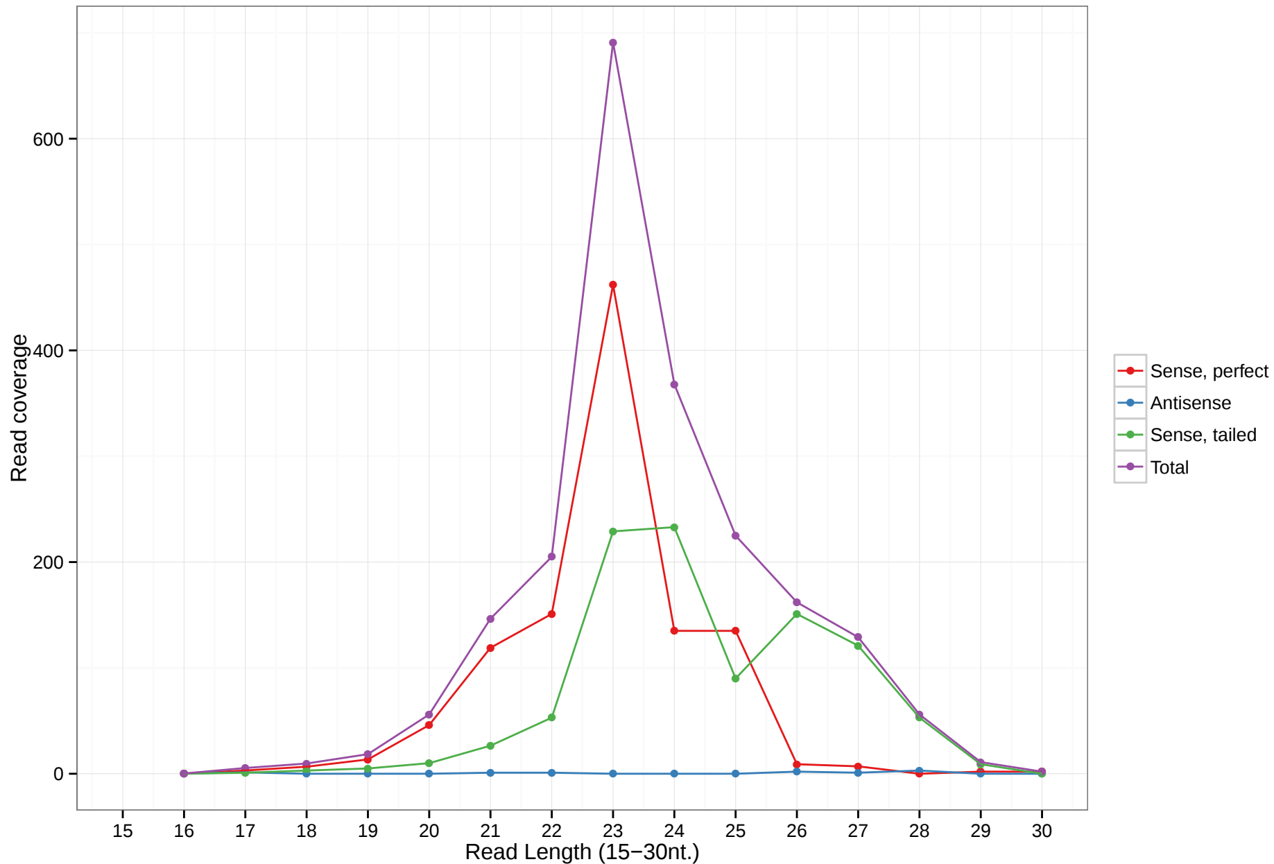
mmu-mir-7049
