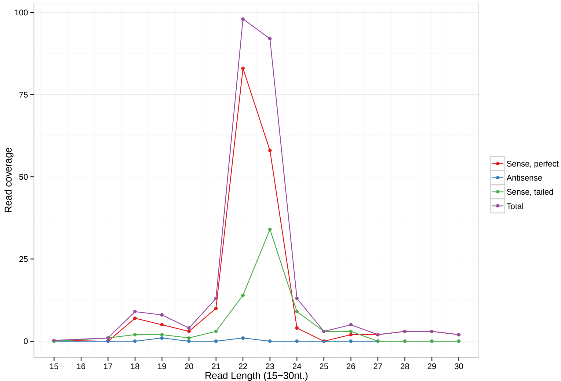
mmu-mir-7048
